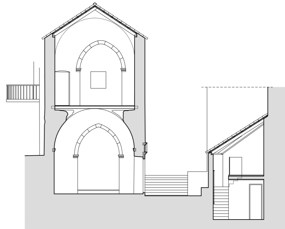
Šibenik, crkva sv. Julijana. Glavni projekt rekonstrukcije i prenamjene. Tlocrt prizemlja (gore) i Presjek 1 (dolje). Izrada: Hrvatski restauratorski zavod, 2020.
