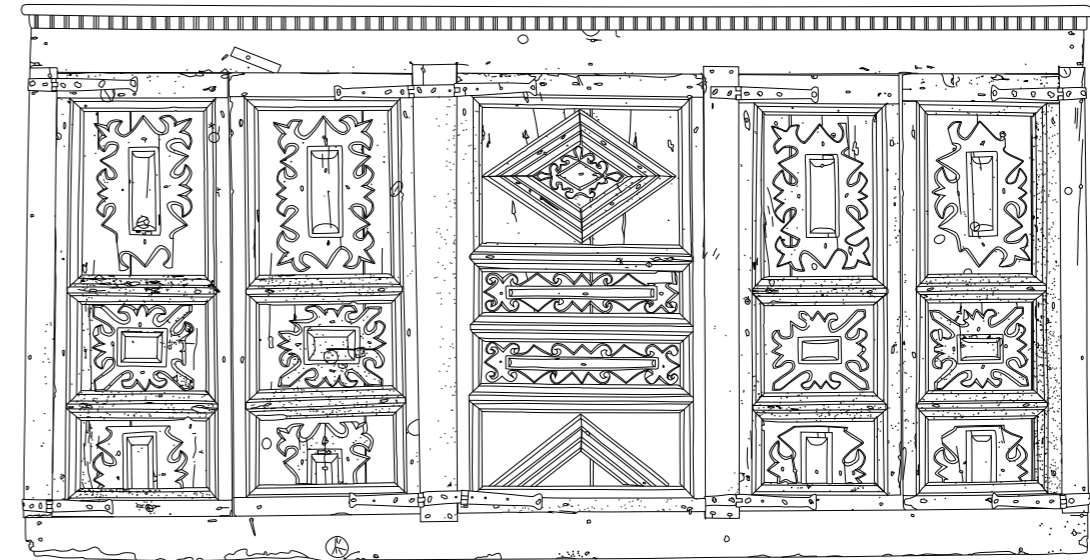
Otok Brač, Škrip, župna crkva sv. Jelene. Nepoznati autor, sakristijski ormar, 15./16. stoljeće. Crtež postojećeg stanja. Izrada: D. Gazde, 2018.
