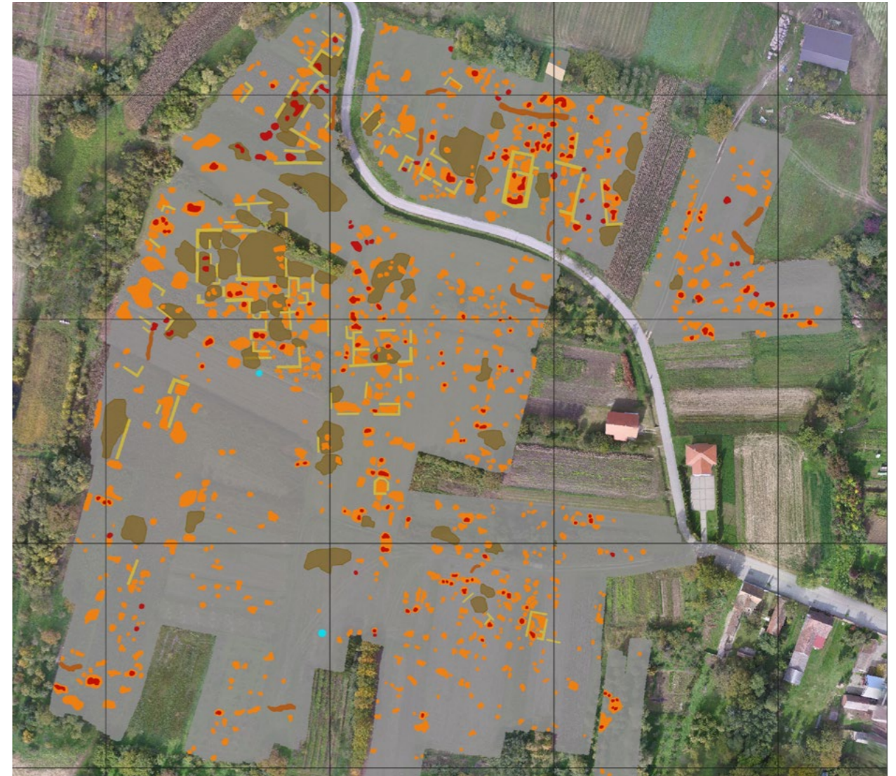
Gorjani – arheološka topografija srednjovjekovnih Gorjana. Rezultati geofizičkog istraživanja. Izrada: Cornelius Meyer Prospection, 2020.
