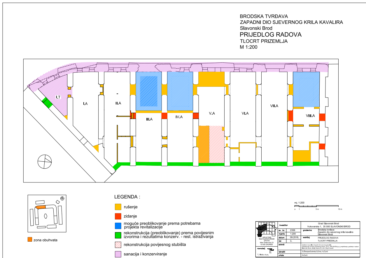
Slavonski Brod, Tvrđava Brod. Sjeverno krilo kavalira, prijedlog radova. Izrada: A. Čurić i D. Škarpa, 2018.
