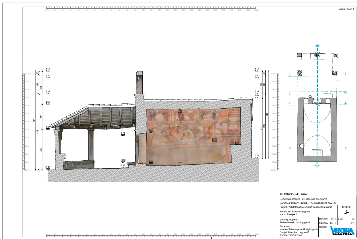
Draguč, crkva sv. Roka. Arhitektonska dokumentacija postojećeg stanja, presjek. Izrada: Vektra, d.o.o., 2018.
