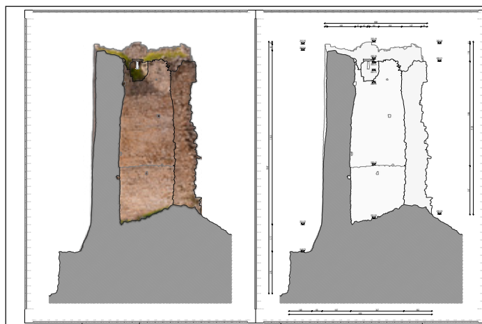
Mokro polje, Keglevića utvrda. Arhitektonska snimka postojećeg stanja – Presjek 7. Izrada: Vektra d.o.o., 2018.
