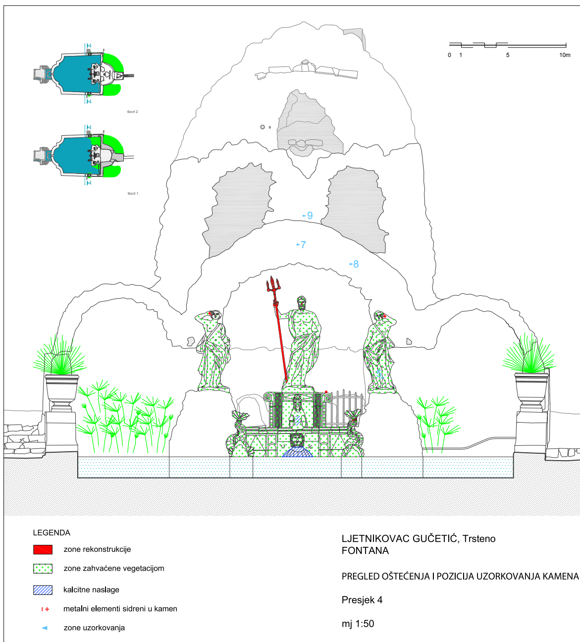
Trsteno, ljetnikovac Gučetić, fontana. Dokumentacija oštećenja. Izrada: V. Marinković, A. Škevin Mikulandra, K. Majer Jurišić, 2018.
