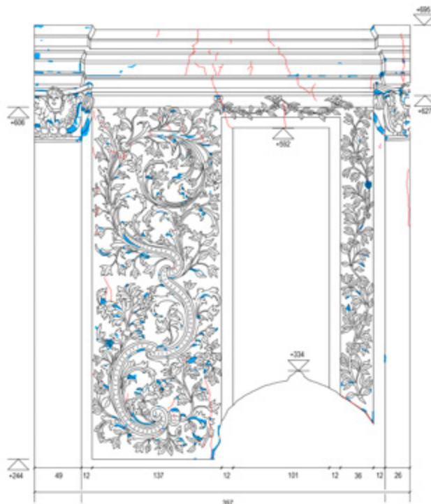
Lepoglava, župna crkva Bezgrešnog začeca Blažene Djevice Marije, kapela Presvetog Trojstva (kapela Patačić), grafički prikaz oštećenja štukature na istočnom zidu. Izrada: T. Rovičanac, 2018.
