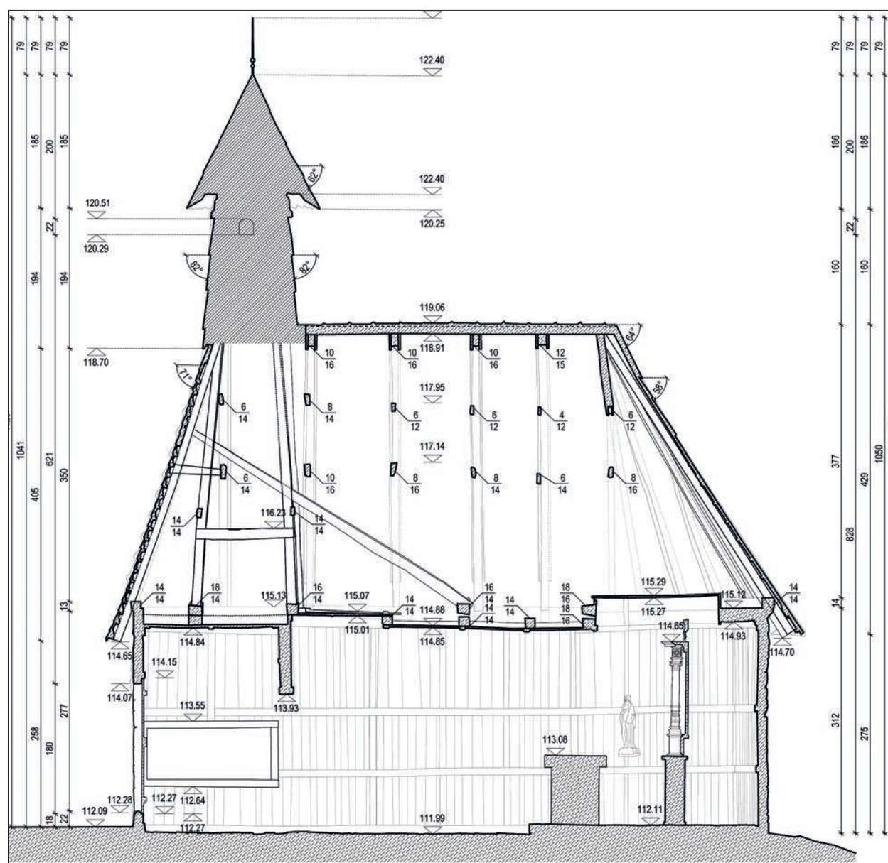
Poljana Lekenička, kapela Sv. Duha i Florijana. Arhitektonski snimak postojećeg stanja – presjek 2-2. Izrada: Vektra d.o.o., 2017.
