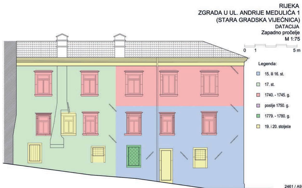
Rijeka, Stara gradska vijećnica. Nacrt zapadnog pročelja s prikazom građevnih faza. Izrada: P. Puhmajer i M. Čalušić, 2017.
