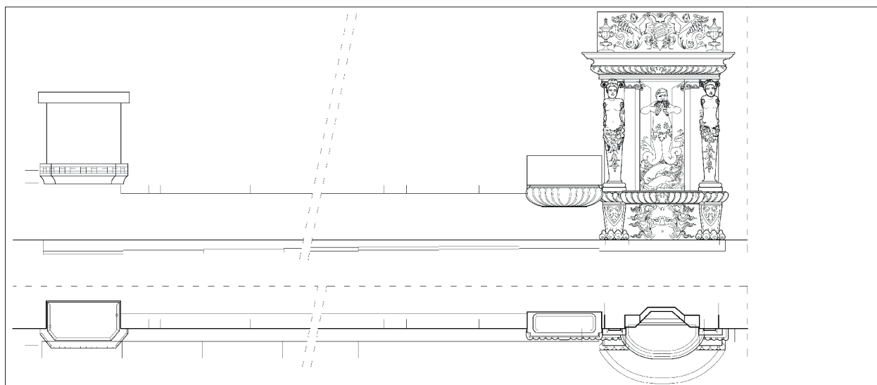
Komolac, ljetnikovac Sorkočević – Skala. Prijedlog rekonstrukcije i prezentacije fontane. Izradila: H. Grebenar, 2017.
