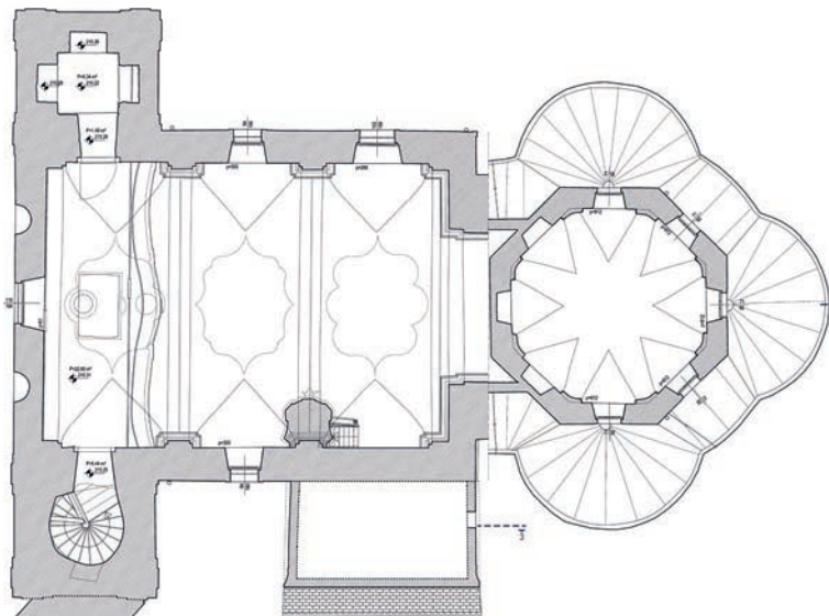
Štrigova, crkva sv. Jeronima. Arhitektonski snimak postojećeg stanja tlocrt pjevališta. Izrada: Vektra d.o.o., 2017.
