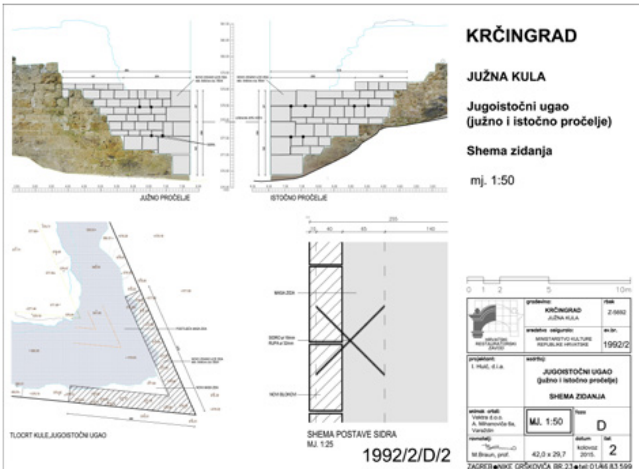
Nacionalni park Plitvička jezera, Krčingrad, južna kula, nacrt sheme zidanja
