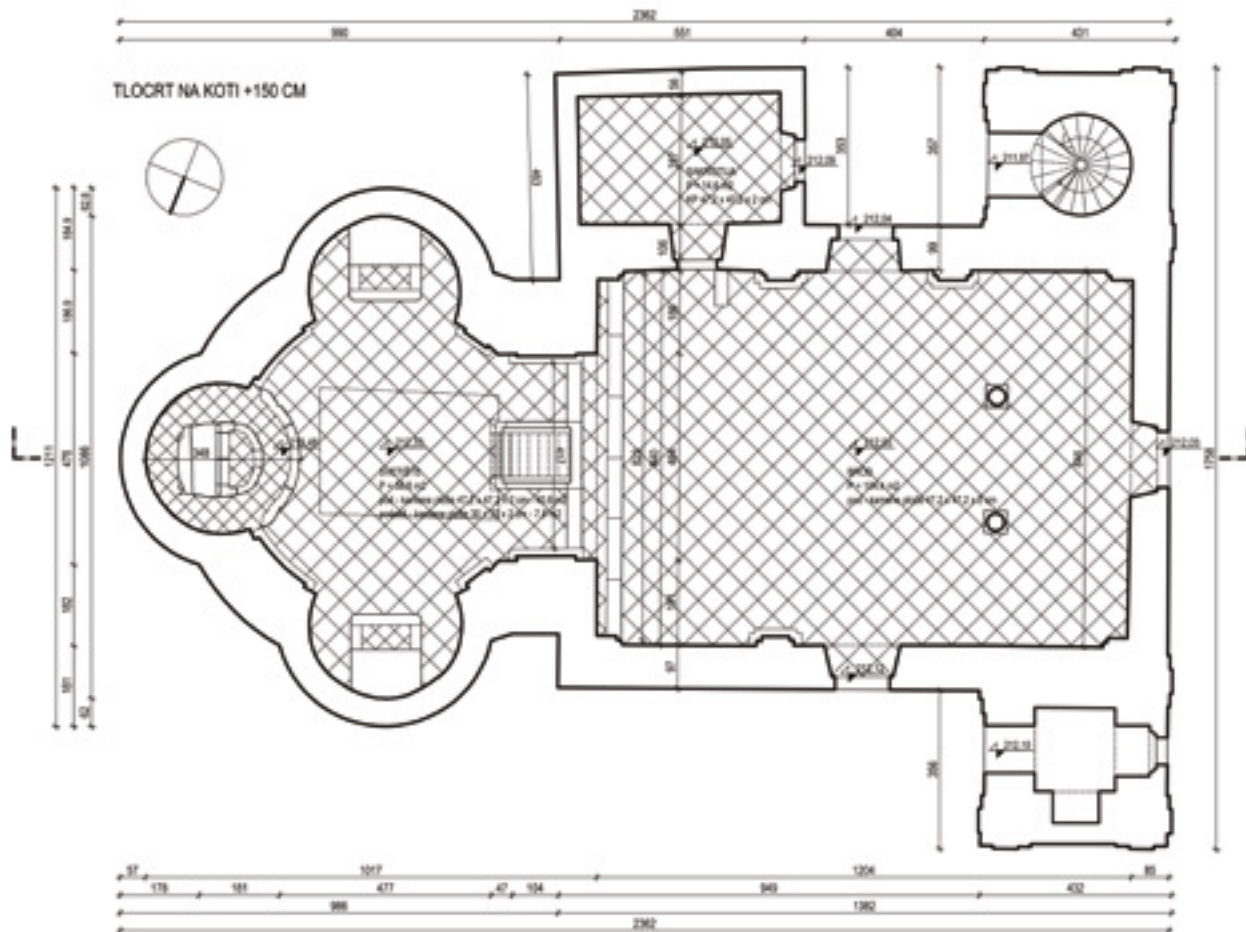
Štrigova, crkva sv. Jeronima, tlocrt - projekt poda
