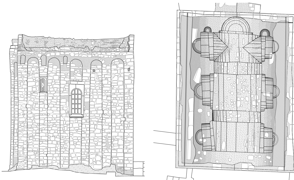
Ston, crkva sv. Mihajla, snimak postojećeg stanja - južno pročelje i tlocrt gornje plohe svoda s evidistancom izvodnica
