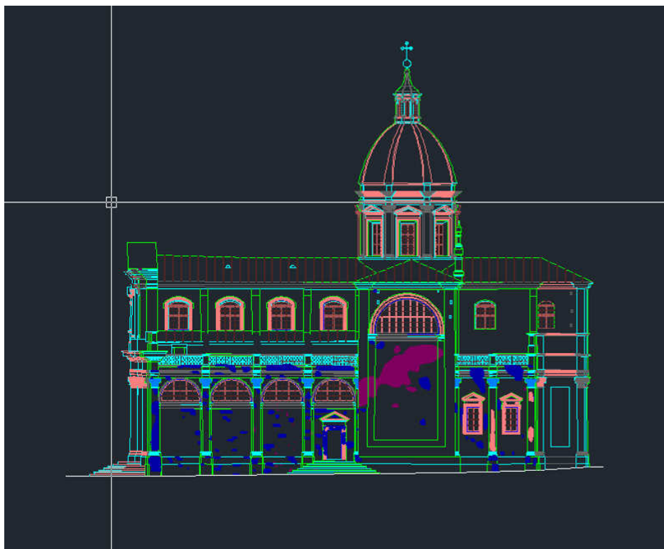
Slika 25. Dubrovnik, katedrala, sjeverno pročelje, mapiranje strukturnih oštećena kamene plastike
