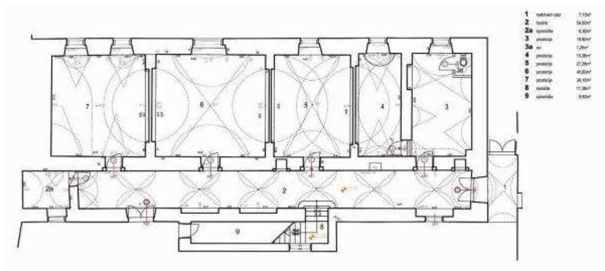
Slika 13. Tlocrt prizemlja krila franjevačkog samostana u kojem je smještena nekadašnja ljekarna
