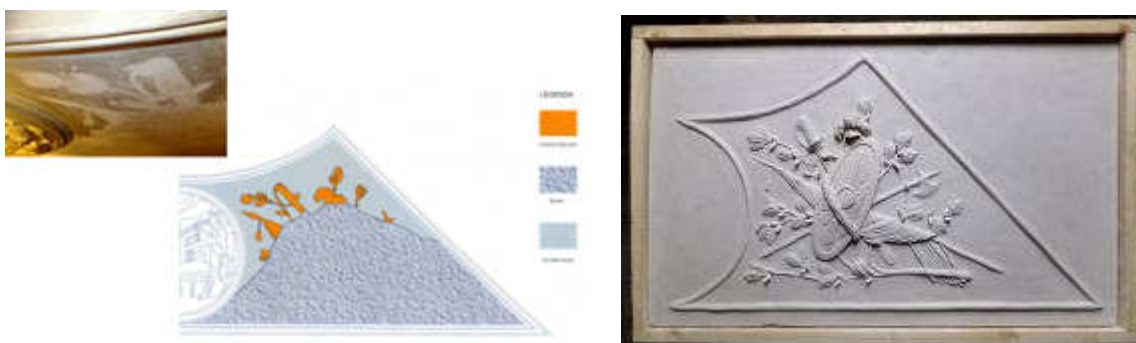
Slika 52. Rijeka, bivša Tvornica šećera, prostorija 18, (slijeva nadesno) stucco ukras u predvorju, detalj nakon uklanjanja preslika; grafički prikaz obrisa nedostajućeg reljefa; model za rekonstrukciju reljefa u MJ 1:25
