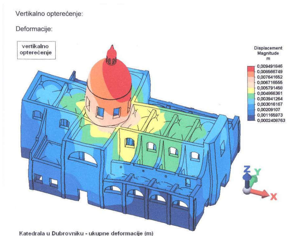
Slika 24. Dubrovnik, katedrala (crkva Uznesenja Marijina), izvadak iz analize postojećeg stanja konstrukcije
