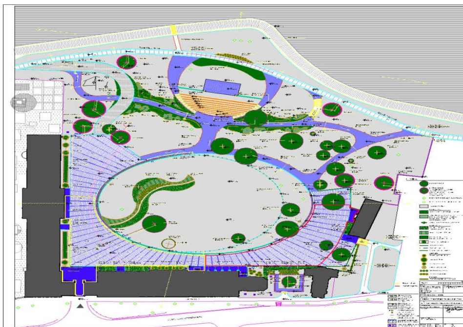
Slika 100. Vukovar, tlocrt Perivoja, crveno obrubljena zona, radovi izvedeni 2013. (Projekt, Arhitektonski fakultet iz Zagreba, projektant dr. sc. S. Jurković, d.i.a., 2010.)
