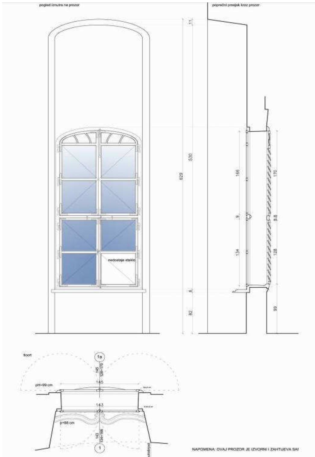
Slika 7. Gornja Bistra, dvorac Oršić, arhitektonska dokumentacija izvornih prozora ovalne dvorane dvorca
