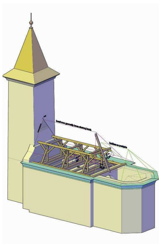
Slika 15. Žumberak, crkva sv. Nikole biskupa, vizualizacija rekonstrukcije krovne plohe na povijesnu visinu
