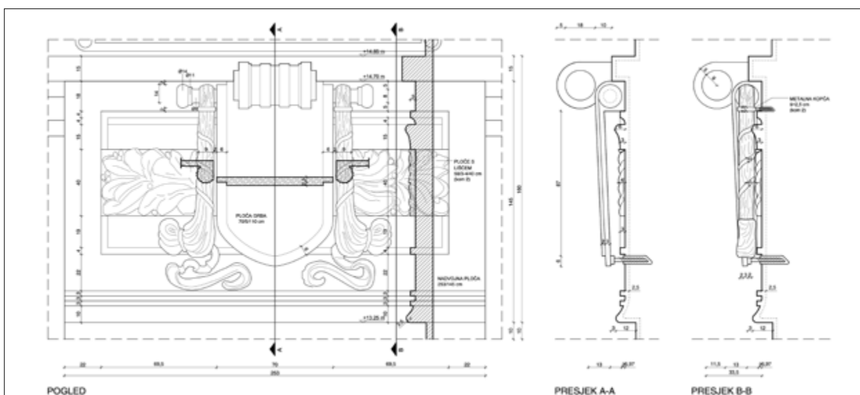
Zagreb, Etnografski muzej. Izvedbeni detalj polja s grbom. Izrada: B. Matica, 2016.
