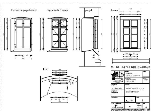
Štrigova, crkva sv. Jeronima. Izvedbeni projekt prozora u svetištu. Izrada: T. Kučinac, 2016.
