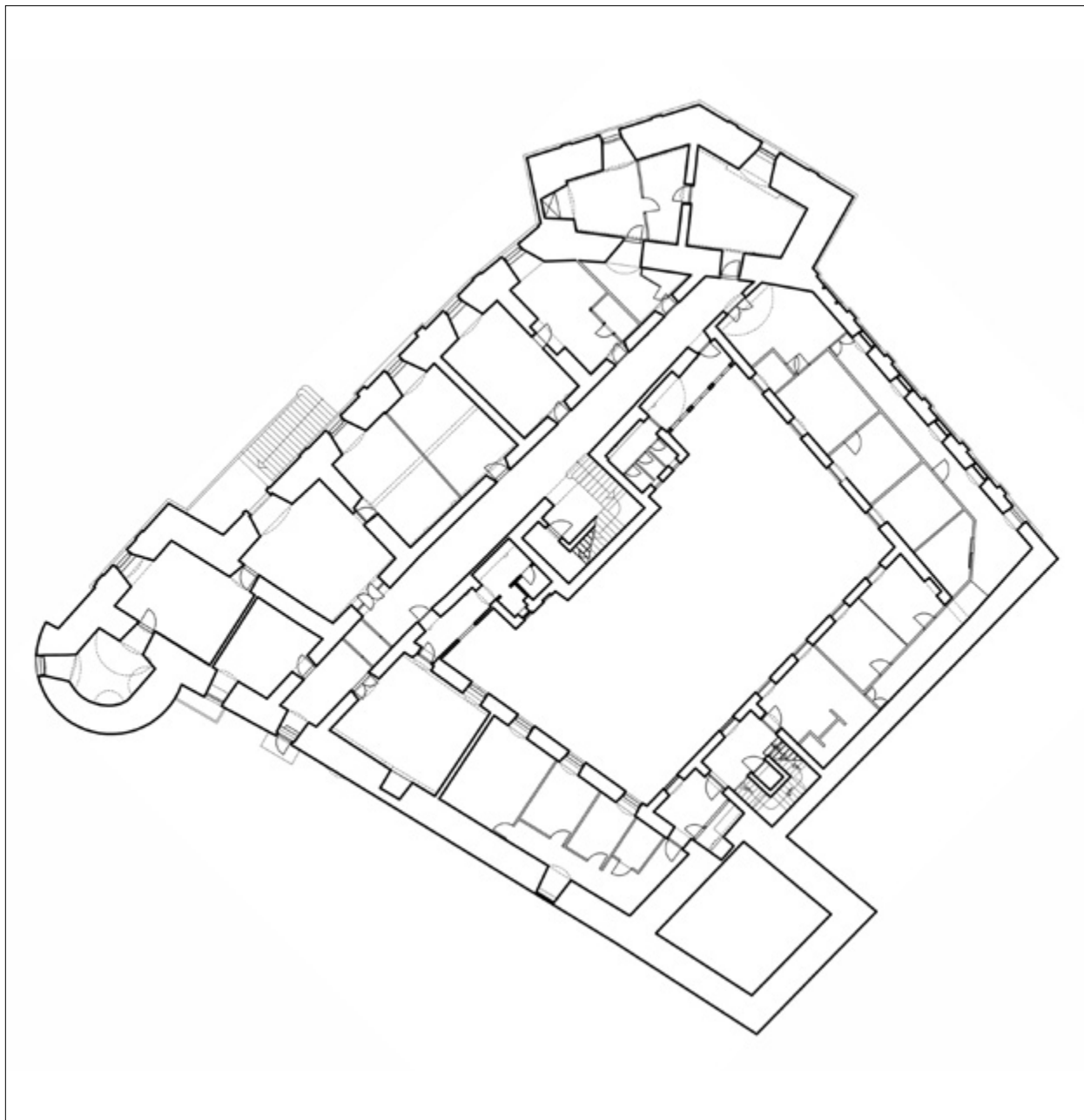
Senj, kaštel Ožegovićanum. Tlocrt prvog kata. Izrada: I. Skomrak, 2016.
