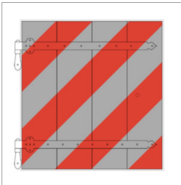
Hum Košnički, Dvor Veliki Tabor. Kula „A“, dvorišno pročelje, poluetaža. Nacrt za rekonstrukciju drvenog kapka prozora iz 16. stoljeća. Izrada: B. Matica, 2016.
